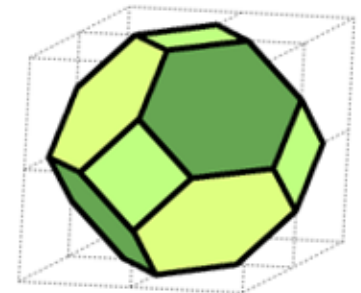
Oktaederstumpf
